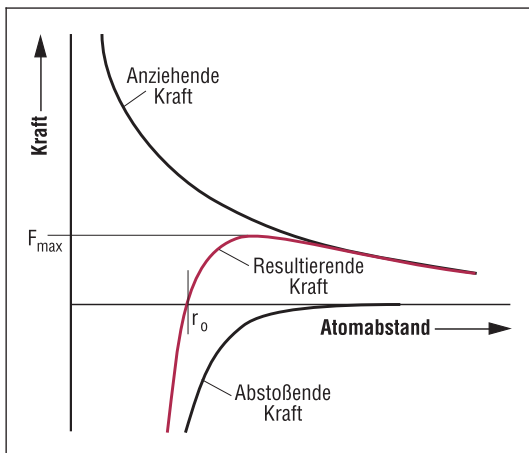
Abb. 2-1: Kräfte im Festkörper
