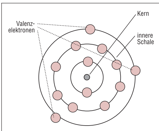
Abb. 2-3: Das Bohrsche Atommodell
