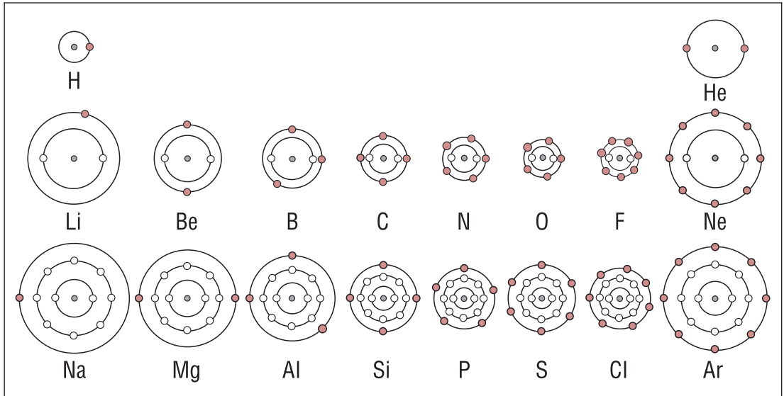
Abb. 2-4: Die Anordnung der ersten 18 Elemente im PSE, gruppiert nach ihrer Valenzelektronenzahl
