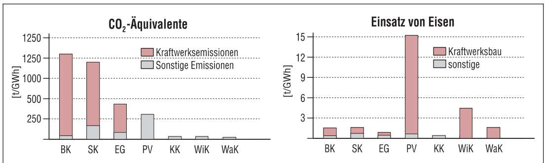
Abb. 6-1: Beispielhafte Resultate für Lebensweganalysen: Treibhausgasemissionen und Aufwand an nicht-energetischen Rohstoffen am Beispiel von Eisen für verschiedene Stromerzeugungstechniken. BK = Braunkohle, SK = Steinkohle, PV = Photovoltaik, KK = Kernkraft, WiK = Windkraft, WaK = Wasserkraft
