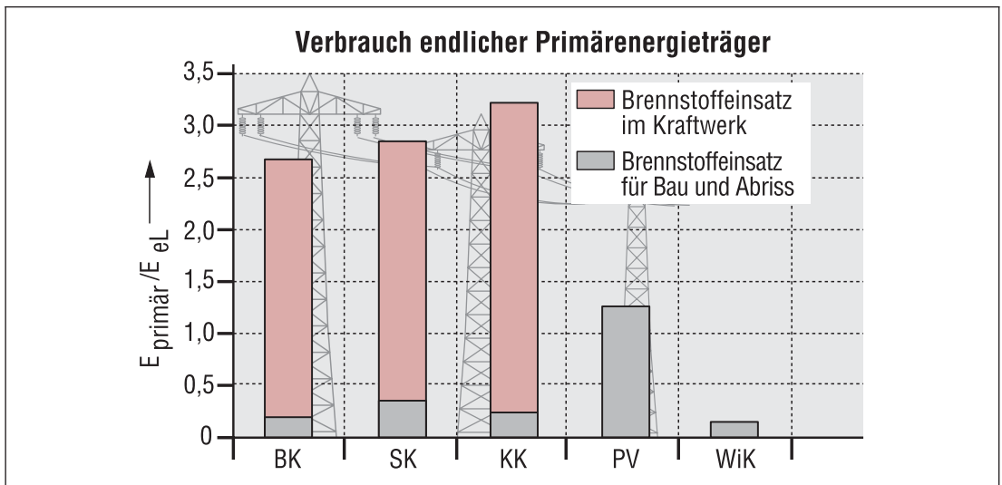
Abb. 6-3: Einsatz an erschöpflicher Primärenergie bei den verschiedenen Stromerzeugungssystemen (BK = Braunkohle, SK = Steinkohle, KK = Kernkraft, PV = Photovoltaik, WiK = Windkraft)
