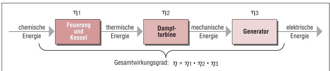
Abb. 3-2: Energiewandlungskette
