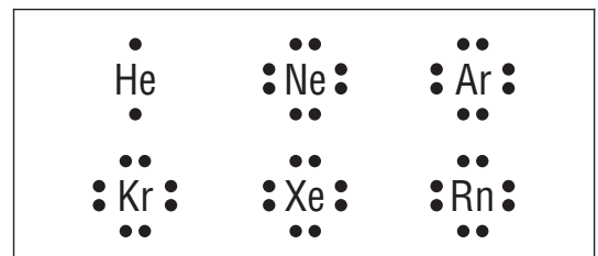
Abb. 2-5: Symbolische Darstellung der Edelgase einschließlich ihrer Valenzelektronen
