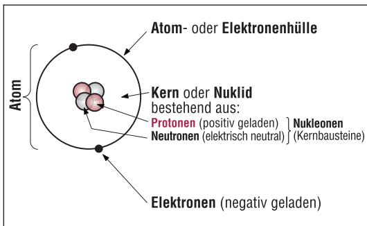
Abb. 5-1: Atommodell zusammen mit den wichtigsten Begriffen, am Beispiel des Heliumatoms
