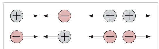
Abb. 2-2: Die Kraftwirkung zwischen elektrisch geladenen Teilchen
